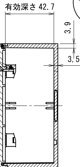
断面 A-A
